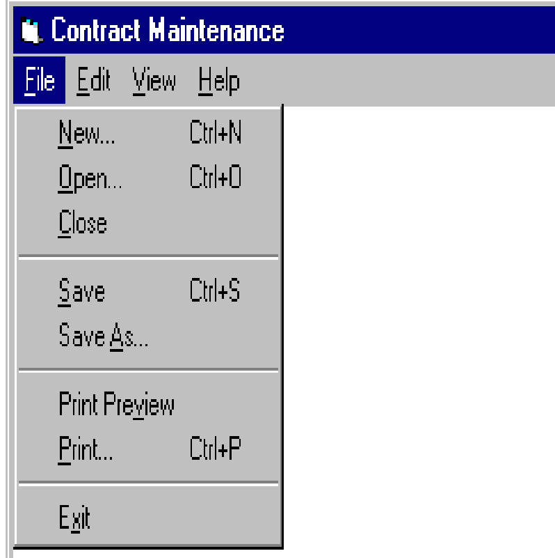
Windows (Arquivo)
