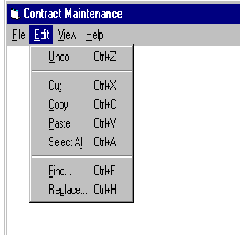
Windows (Editar)
