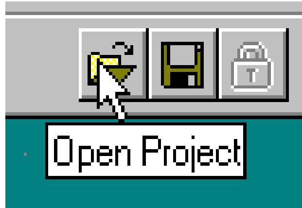
Tooltip
